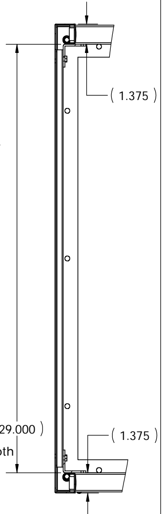
SECTION B-B SCALE 1 : 6
